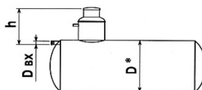
Горизонтальная установка
